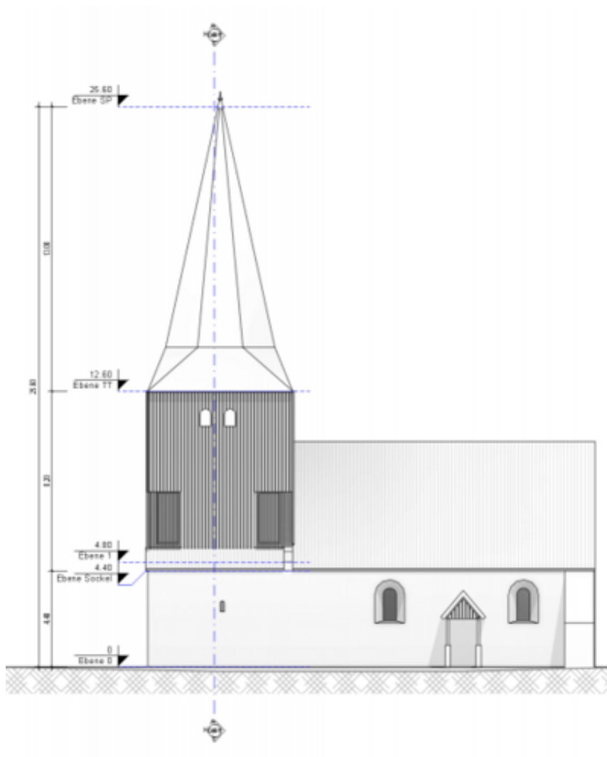
Seitenansicht Kirche Rosenhagen
