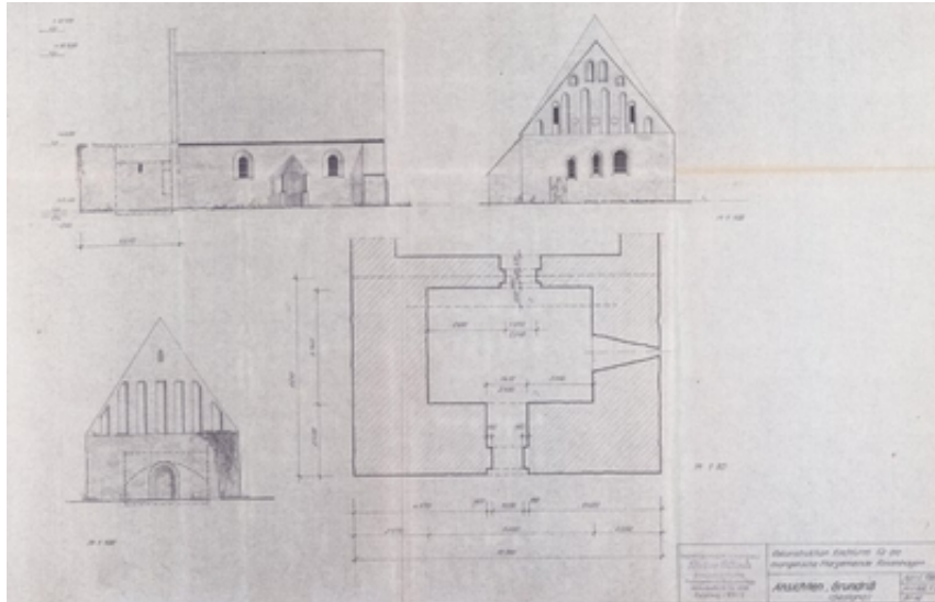
Maßskizze Kirche Rosenhagen
